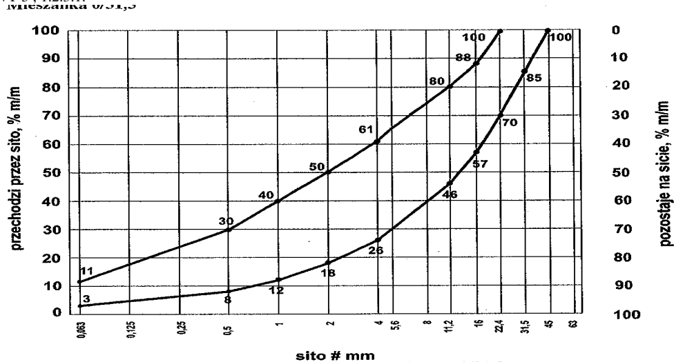
Rys. 1.1. Uziarnienie mieszanki CBGM 0/31,5
