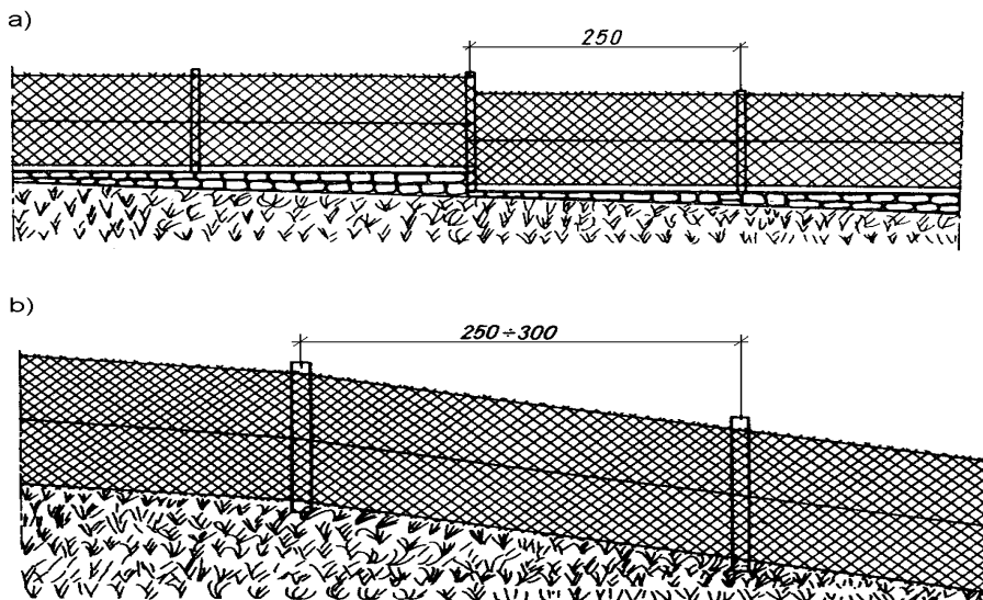
Rys. 6. Przykład ustawienia ogrodzenia siatkowego na terenie pochyłym (wg [6]) a) Ogrodzenie ze stopniami wysokości 25÷30 cm (przy spadku terenu od 1:16 do 1:30) b) Ogrodzenie równoległe do terenu
