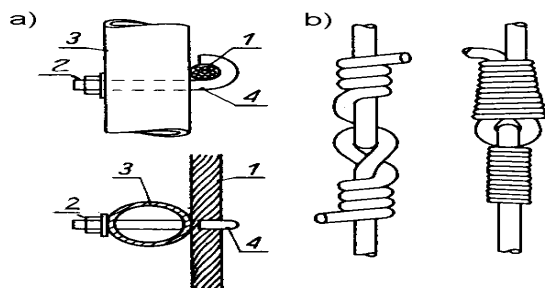
Rys. 8. Przykład napinania siatki przy ustawianiu ogrodzenia (wg [6])
