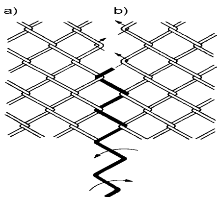
Rys. 2. Łączenie dwóch sąsiednich odcinków siatki za pomocą spirali wyplecionej z siatki i wprowadzonej w oczka siatki ruchem śrubowym (wg [6])
