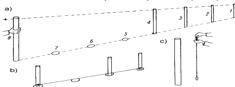
Rys. 4. Przykład ustawiania słupków ogrodzenia (wg [6])
