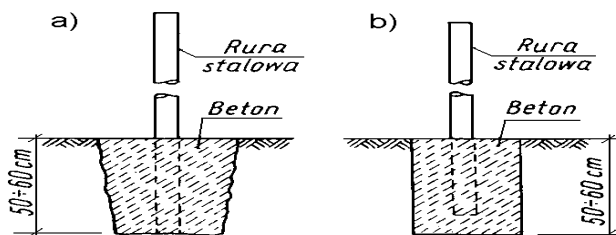
Rys. 4. Przykład ustawiania słupków ogrodzenia (wg [6])
