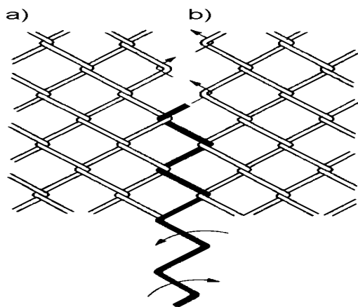
Rys. 2. Łączenie dwóch sąsiednich odcinków siatki za pomocą spirali wyplecionej z siatki i wprowadzonej w oczka siatki ruchem śrubowym (wg [6])
